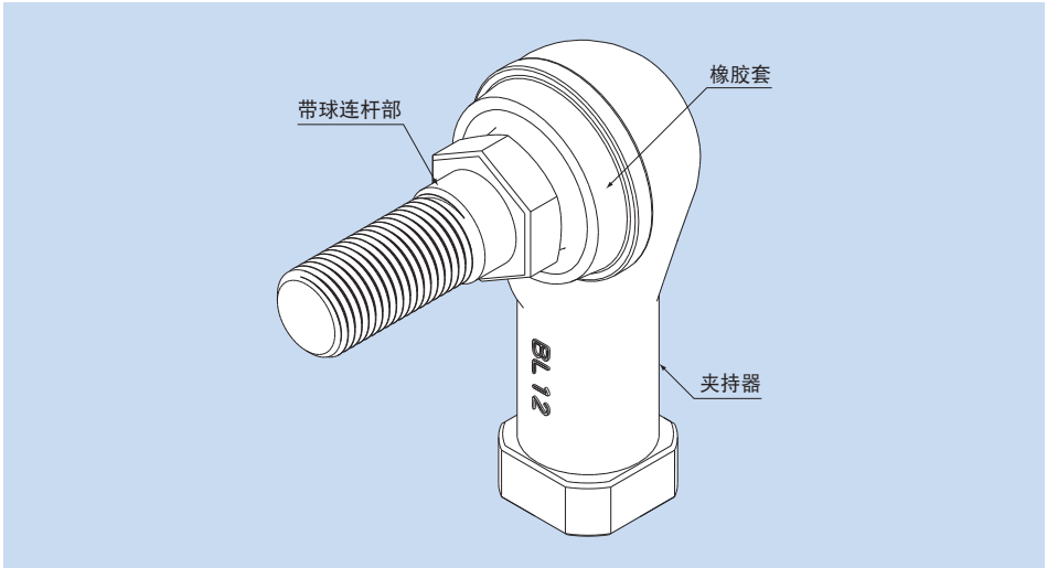
图1 杆端球面接头BL型的结构
