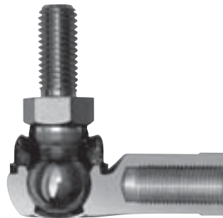
BL型球面部切割样本
